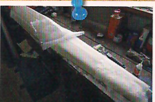
19 - La demi-coque en balsa a été posée sur les couches de tissu imprégnées, et maintenant, on pose la couche de tissu de verre extérieure. Ainsi, on va obtenir un «sandwich» fibre-balsa-fibre, ultra léger et aussi très résistant. Les premiers planeurs «grandeur» en fibre étaient réalisés ainsi.
