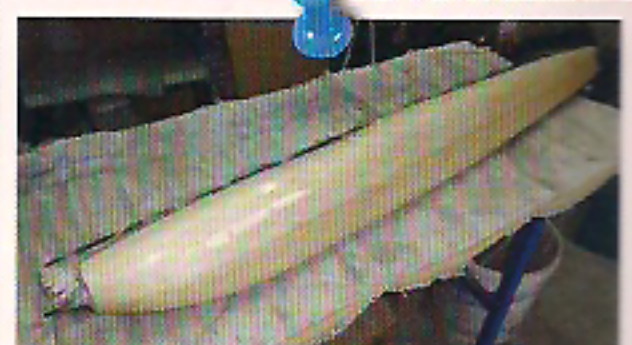
23 - Il reste à attendre le durcissement de la résine avant de pouvoir sortir une demi-coque stratifiée de son moule.
