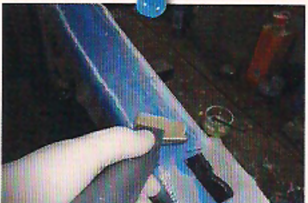
18 - Les couches de fibre sont imprégnées de résine époxy avec un petit rouleau en mousse.
